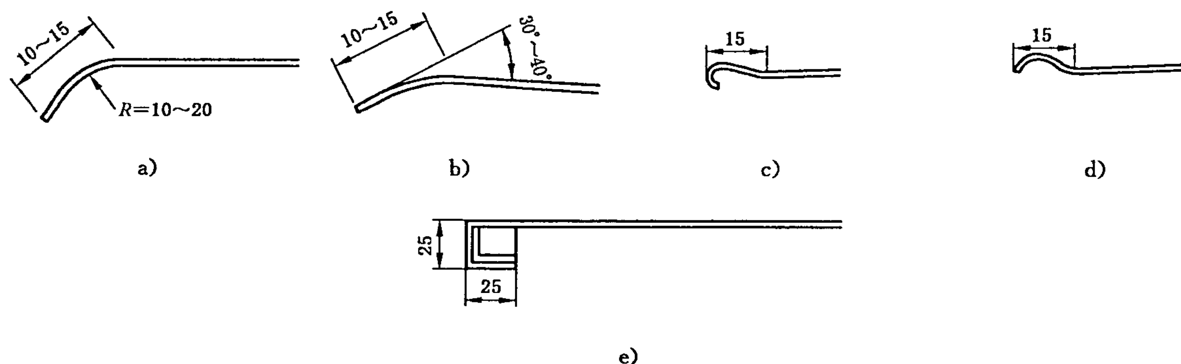
图 1 标志板卷边型式
