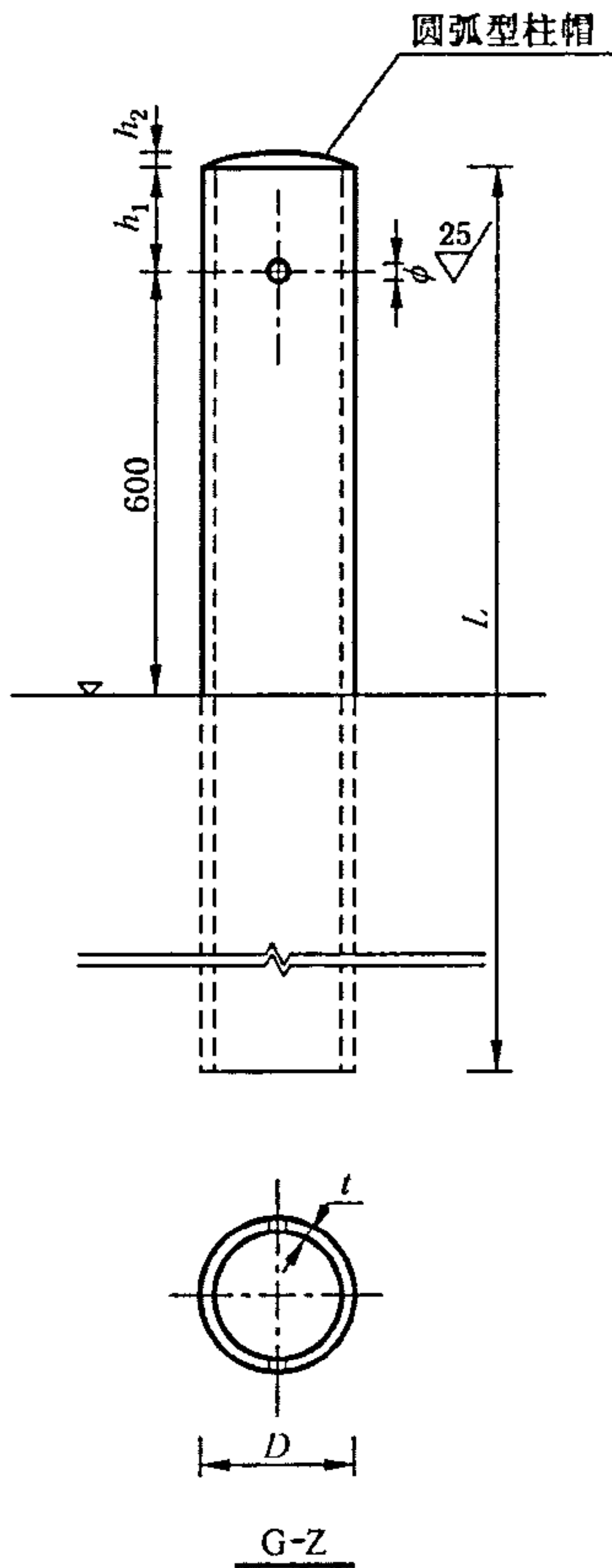
图 7 立柱
