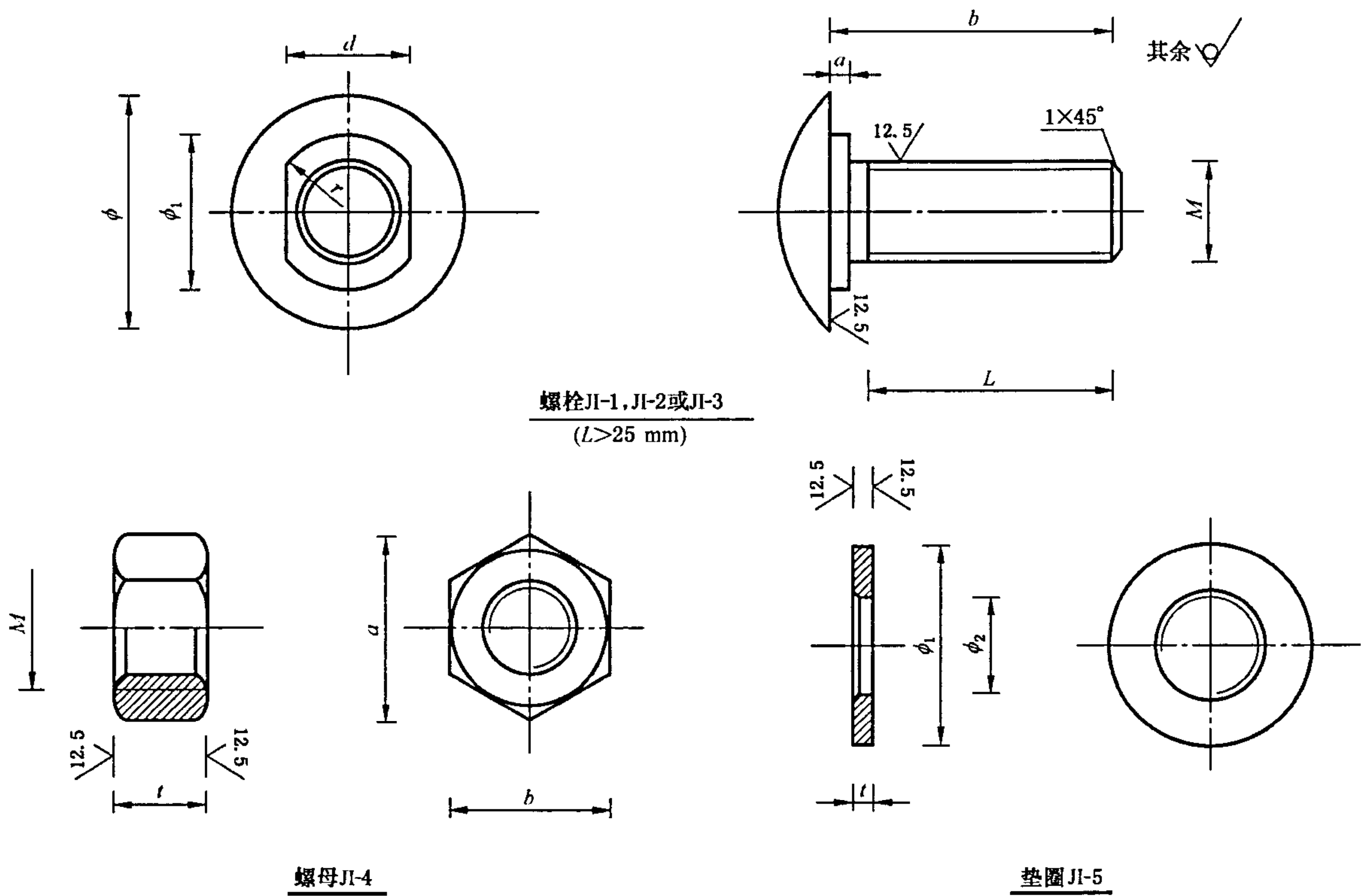
图 10 拼接螺栓
