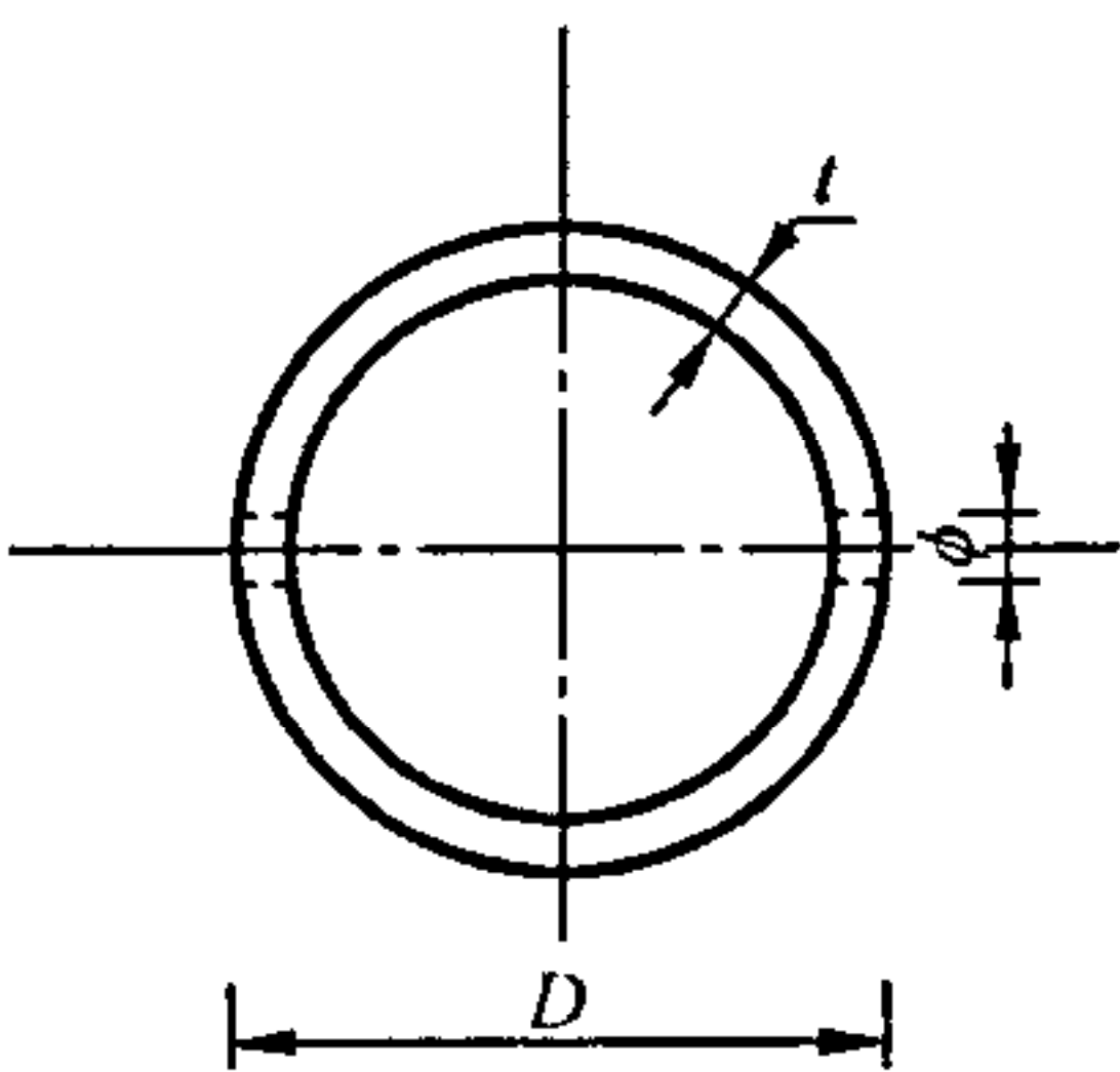
图 6 立柱断面形状
