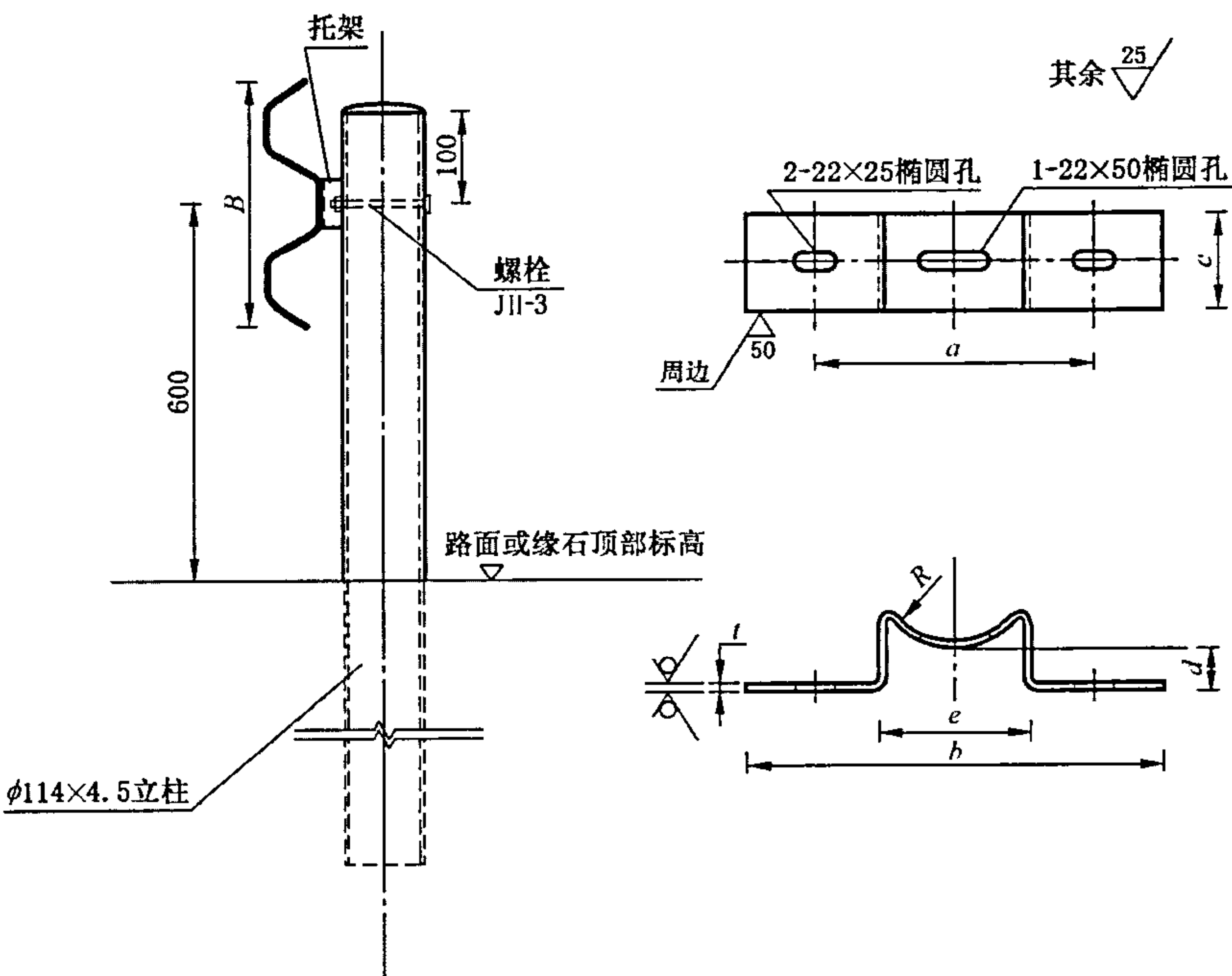
图 13 托架
