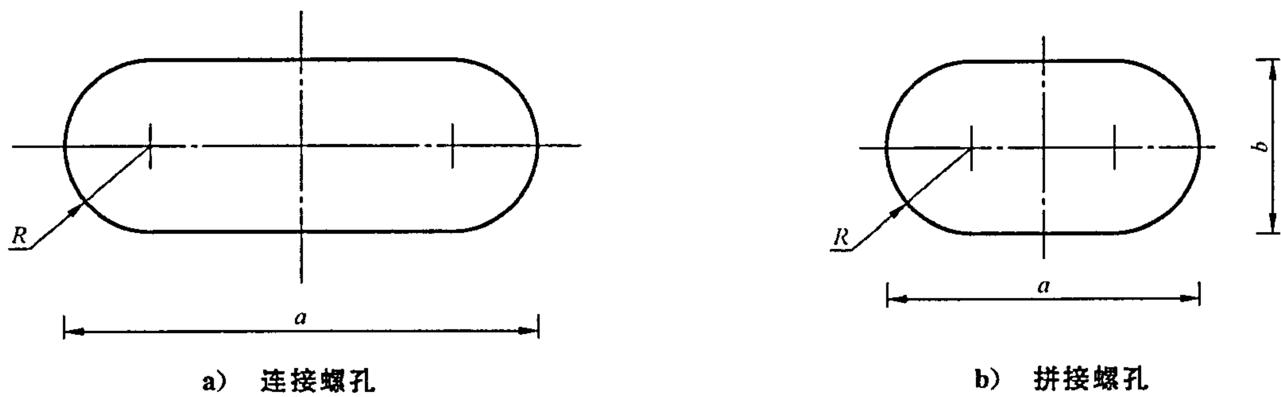
图 5 螺孔尺寸
