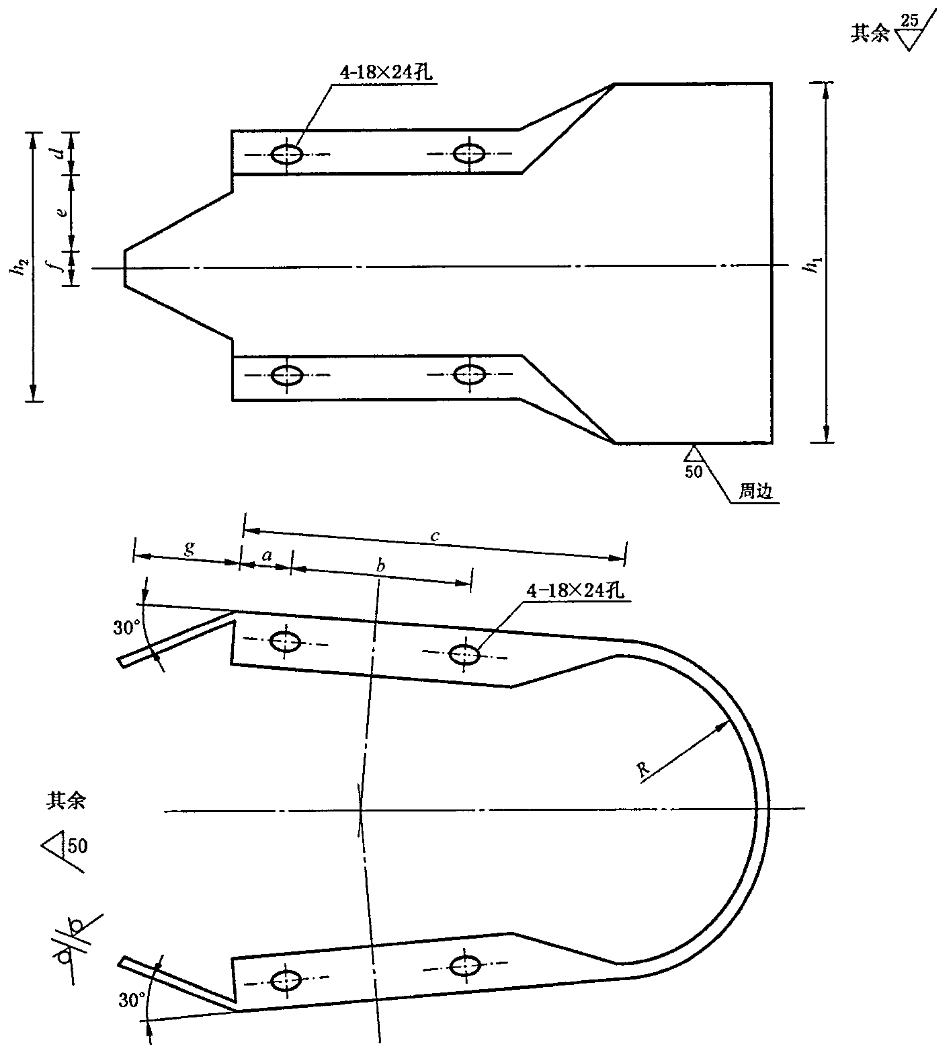
图 9 端头(D-II 或 D-III)
