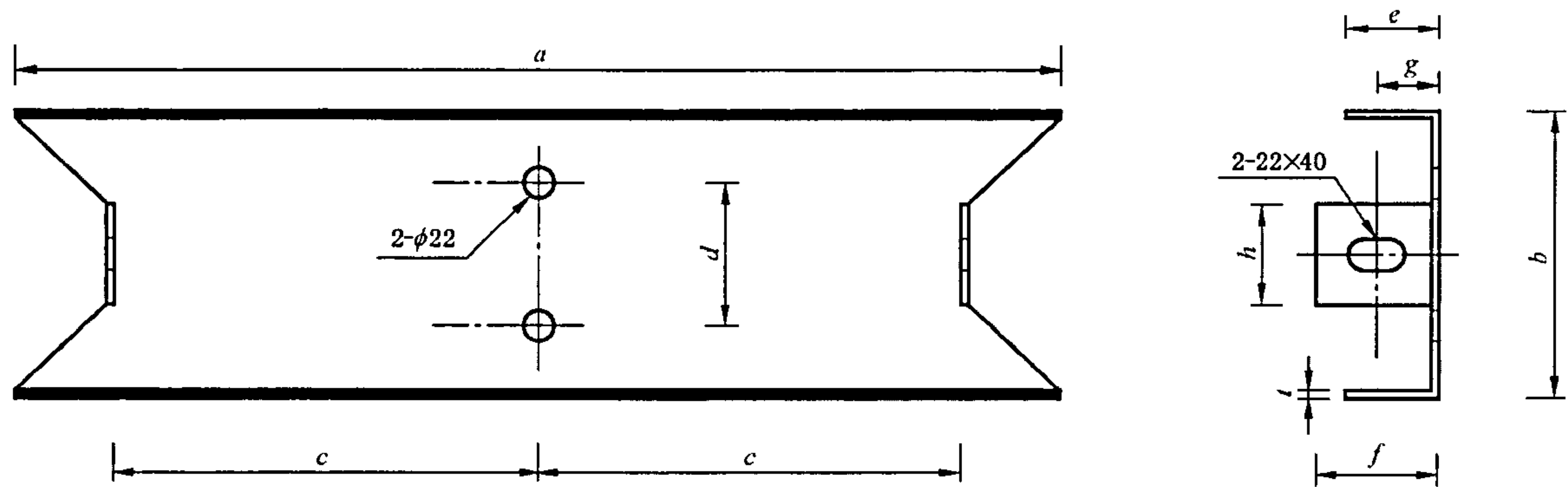
图 14 横隔梁
