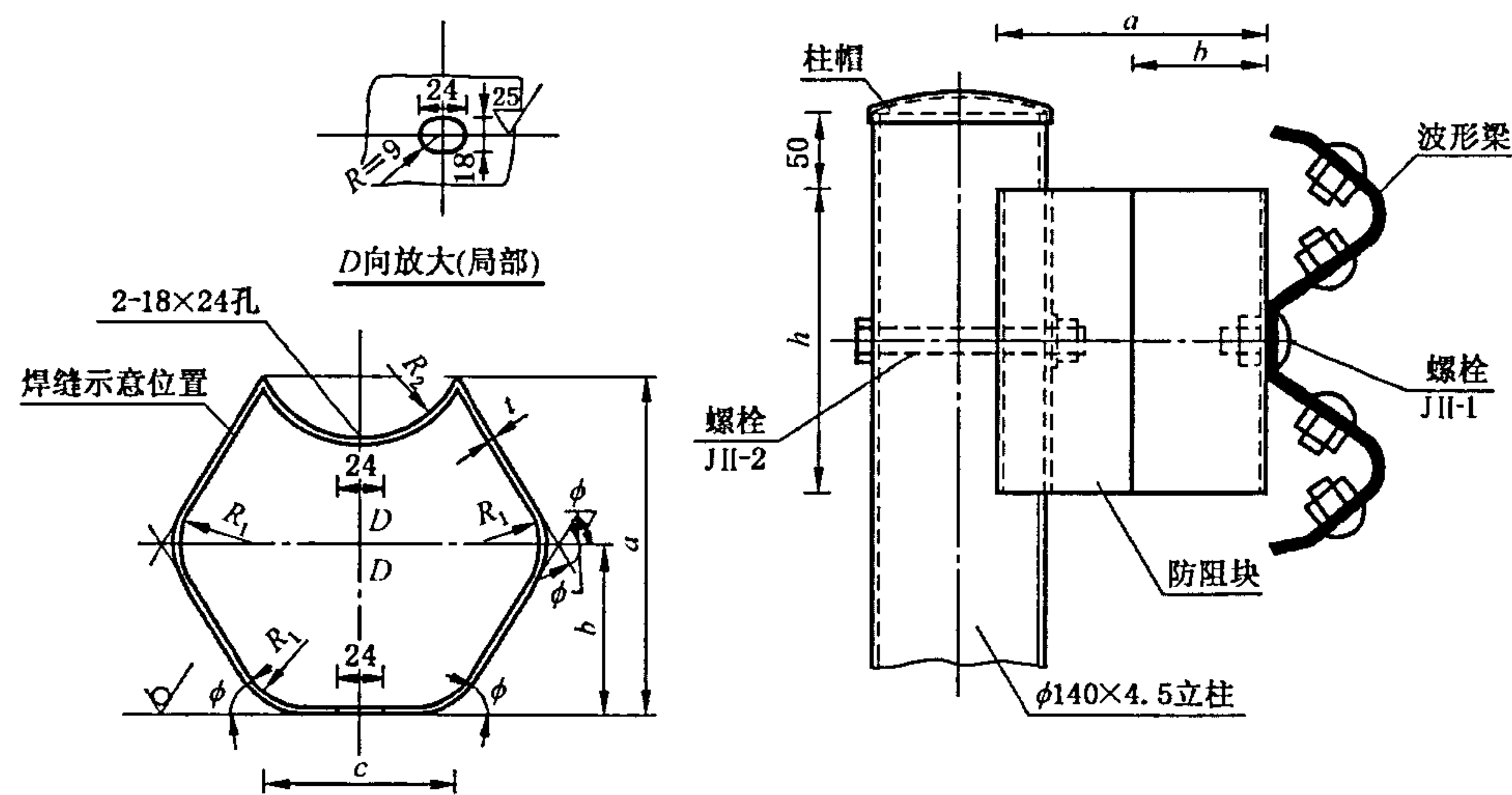
图 12 防阻块
