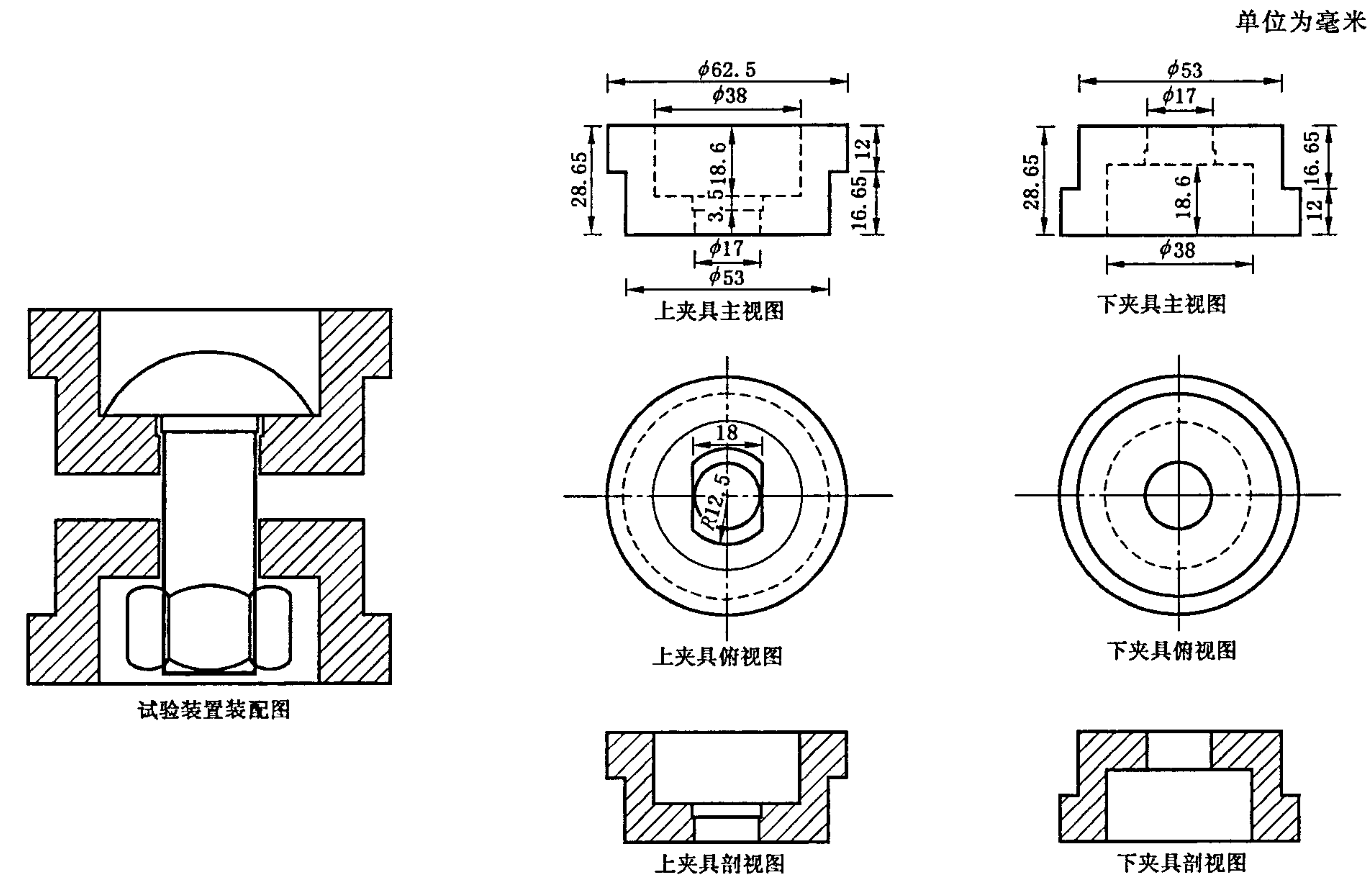
图 A.1 抗拉荷载试验装置图
