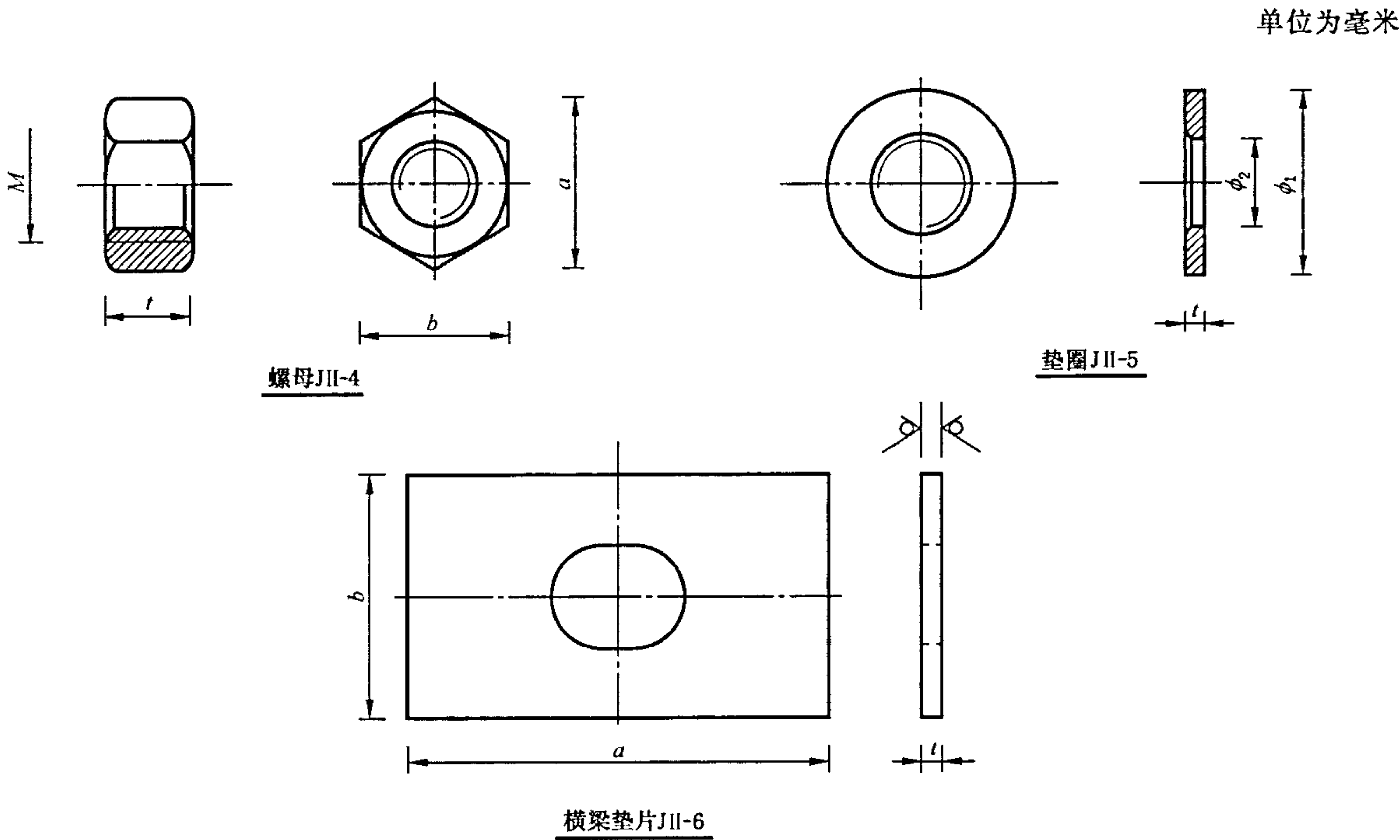
图 11 连接螺栓和横梁垫片
