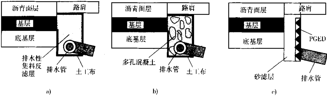
图 10-1 AASHTO 沥青路面结构层边缘排水方案 a)类型 A;b)类型 B;c)类型 C
