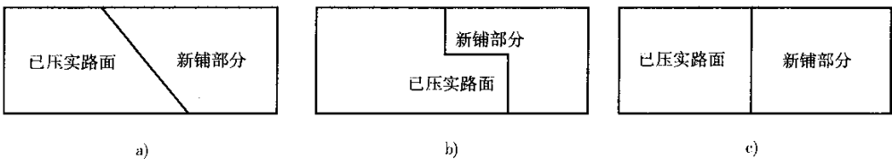
图 5.8.3 横向接缝的几种型式
