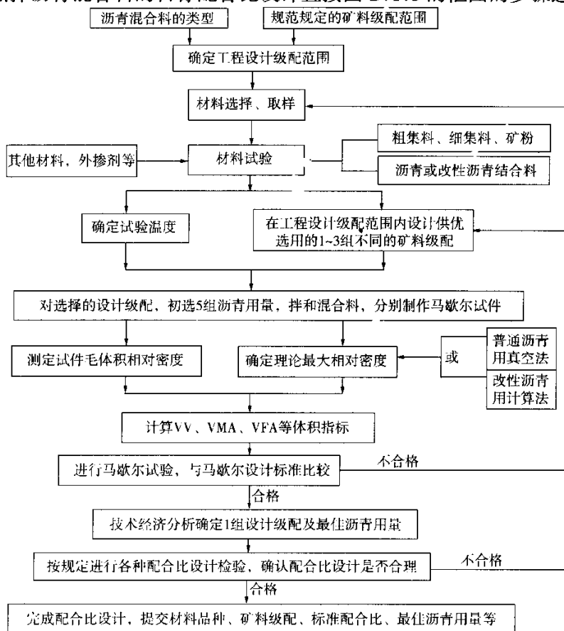
图 B.1.3 密级配沥青混合料目标配合比设计流程图
