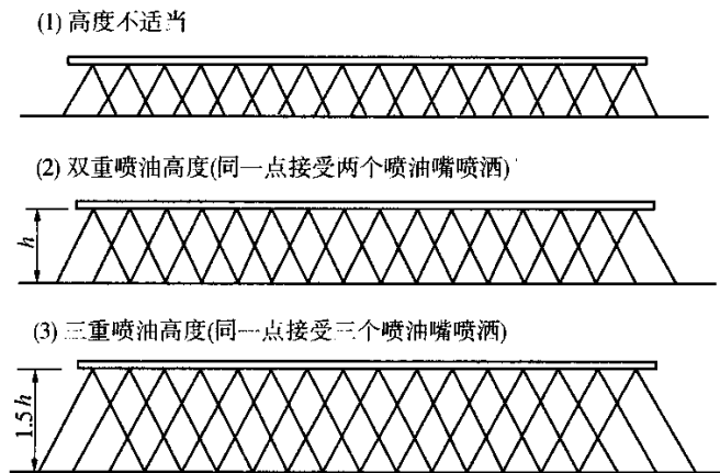
图 6-1 沥青洒布车喷油嘴的高度
