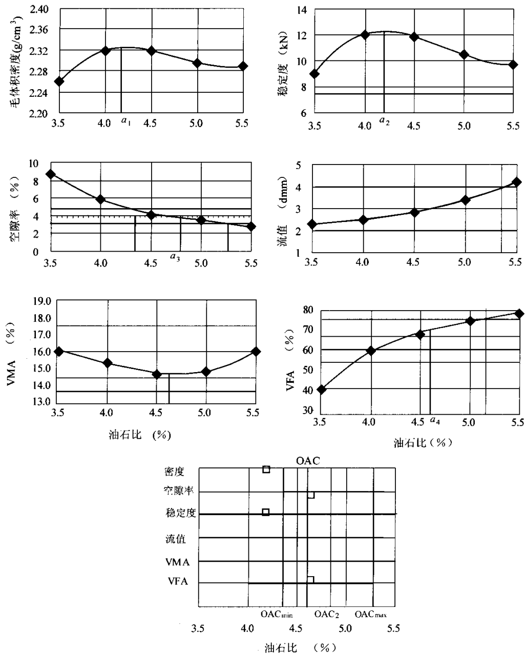
图 B.6.1 马歇尔试验结果示例
