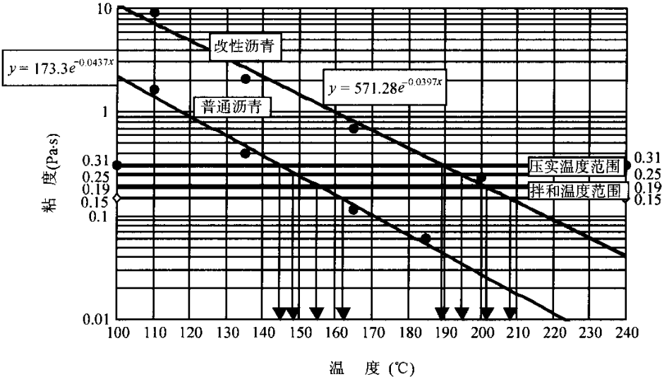
图 5-1 普通沥青及改性沥青的粘温曲线
