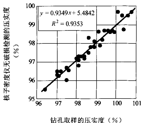
图 11-1 核子仪与钻孔试件结果的标定关系
