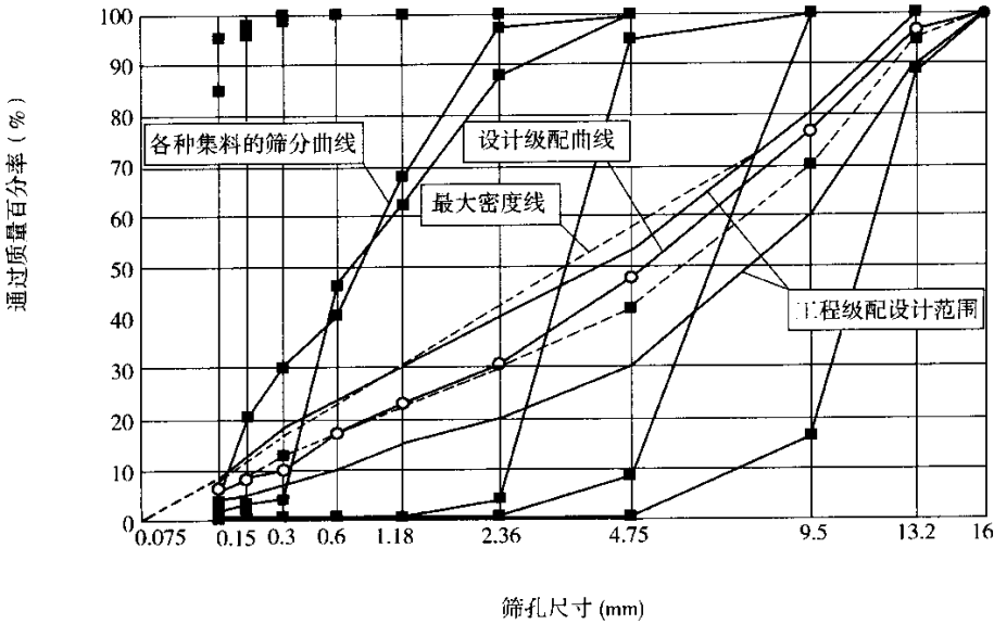
图 B.4.2 矿料级配曲线示例
