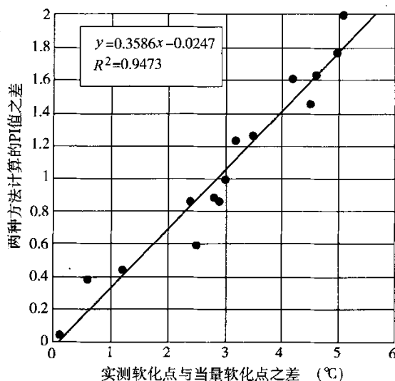
图 4-1 不同软化点测定方法与 PI 值计算结果的关系
