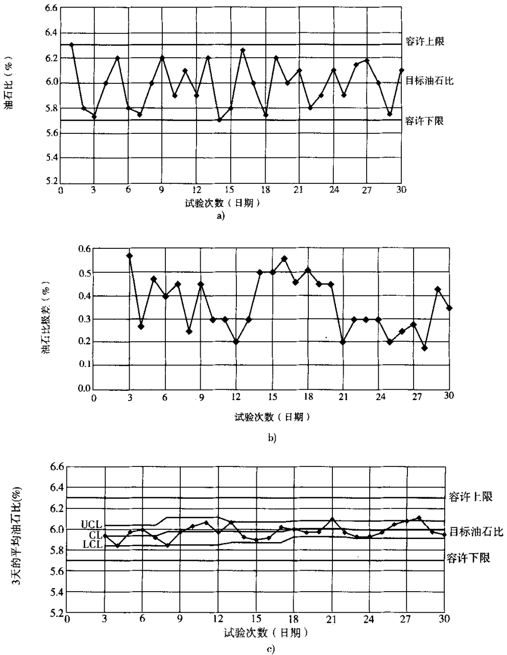
图 F-2 动态质量管理图( \bar{x}-R 管理图)示例(油石比, %)
