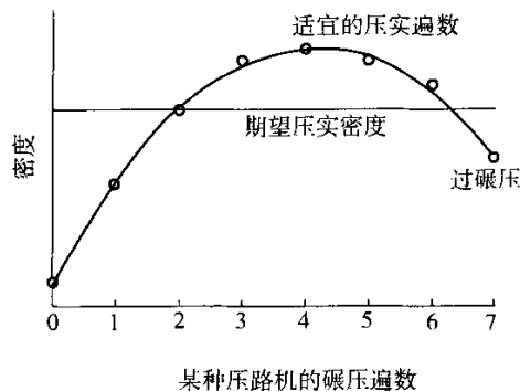
图 11-2 沥青路面的过碾压
