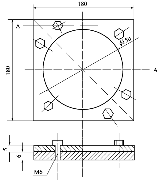
图 7 流动度制样器示意图
