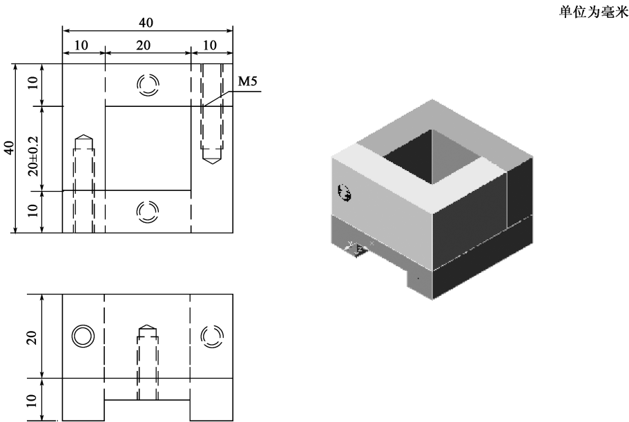
图 4 热熔型涂料密度制样器示意图
